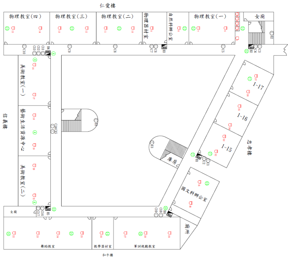
文華高中科學樓3F消防設備平面圖
