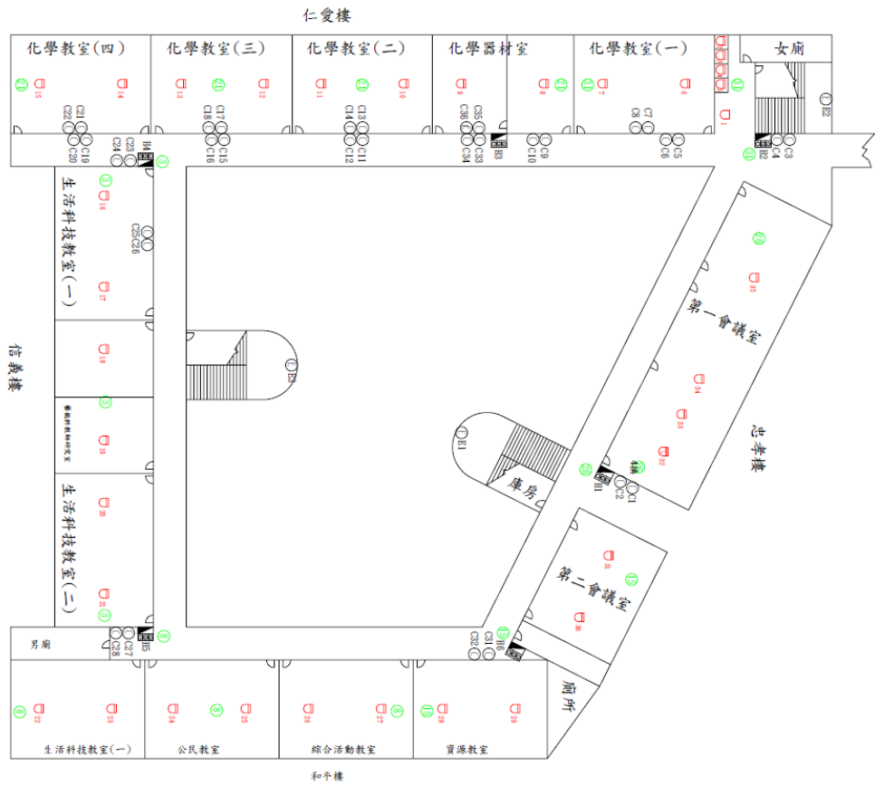
文華高中科學樓2F消防設備平面圖
