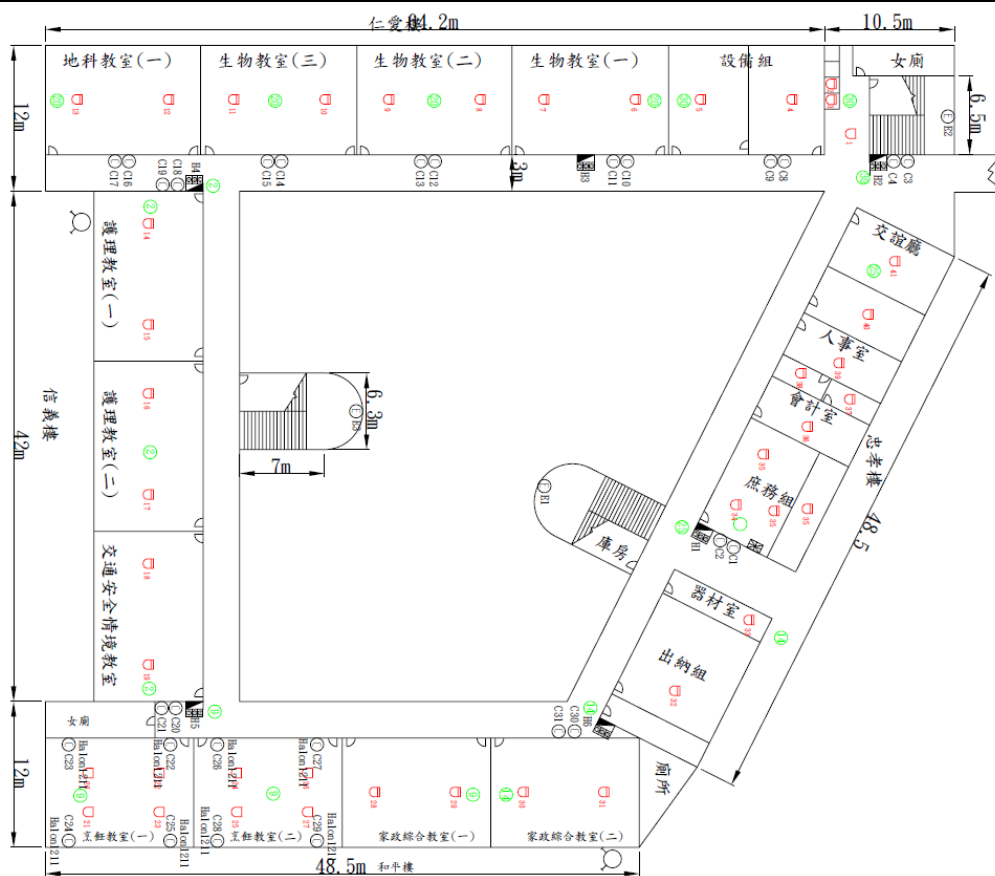
文華高中科學樓1F消防設備平面圖
