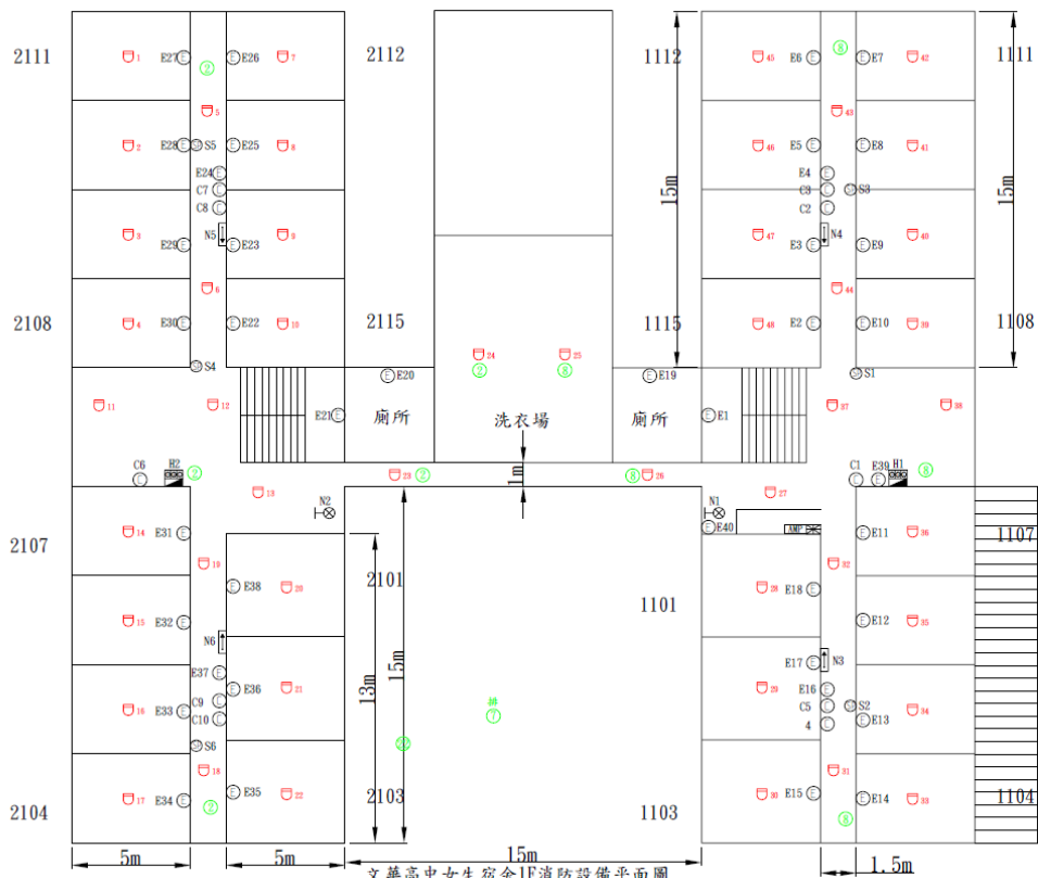
文華高中女生宿舍B1F消防設備平面圖
