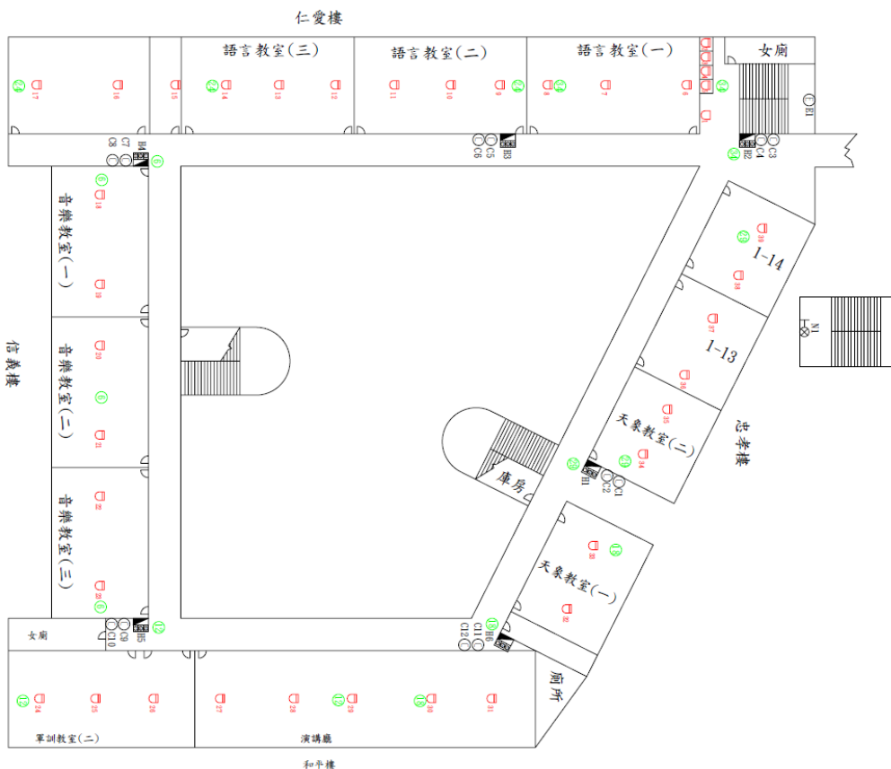
文華高中科學樓5F消防設備平面圖
