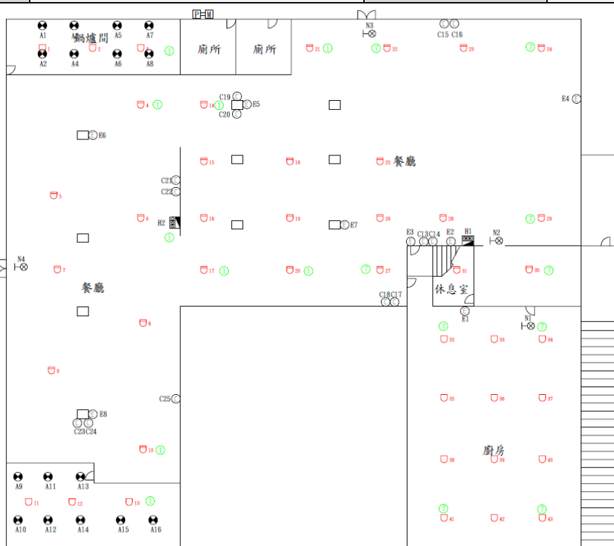
文華高中女生宿舍B1F消防設備平面圖
